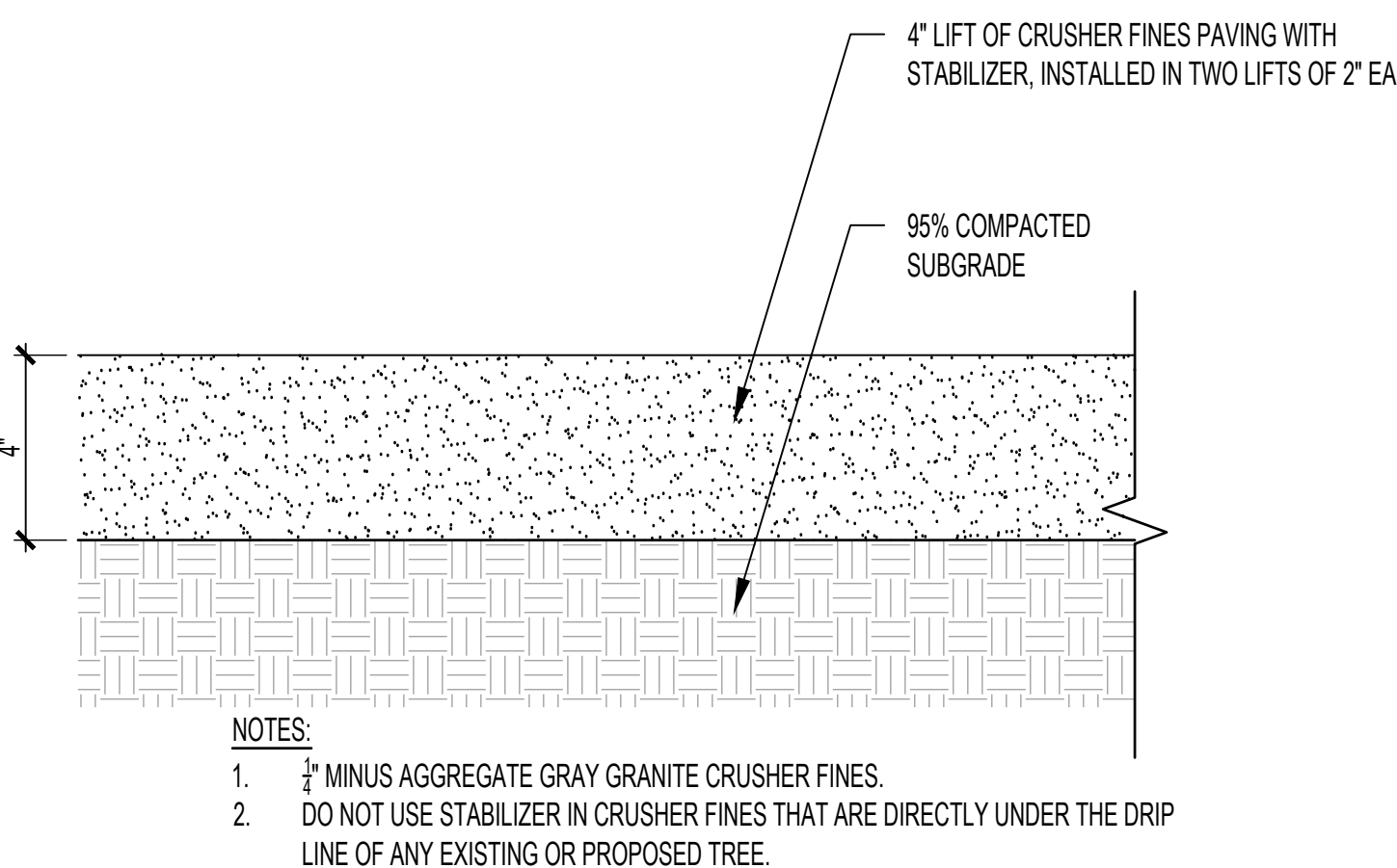
B CRUSHER FINES SCALE: 3/4" = 1'-0"
