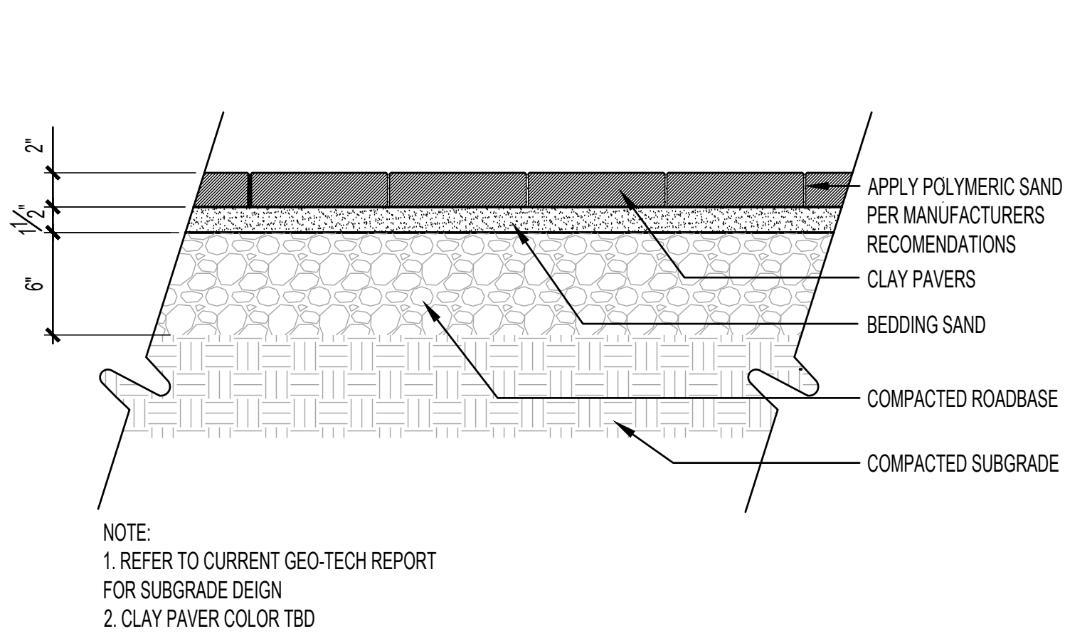
A CLAY PAVERS SCALE: 1/12" = 1'-0"
