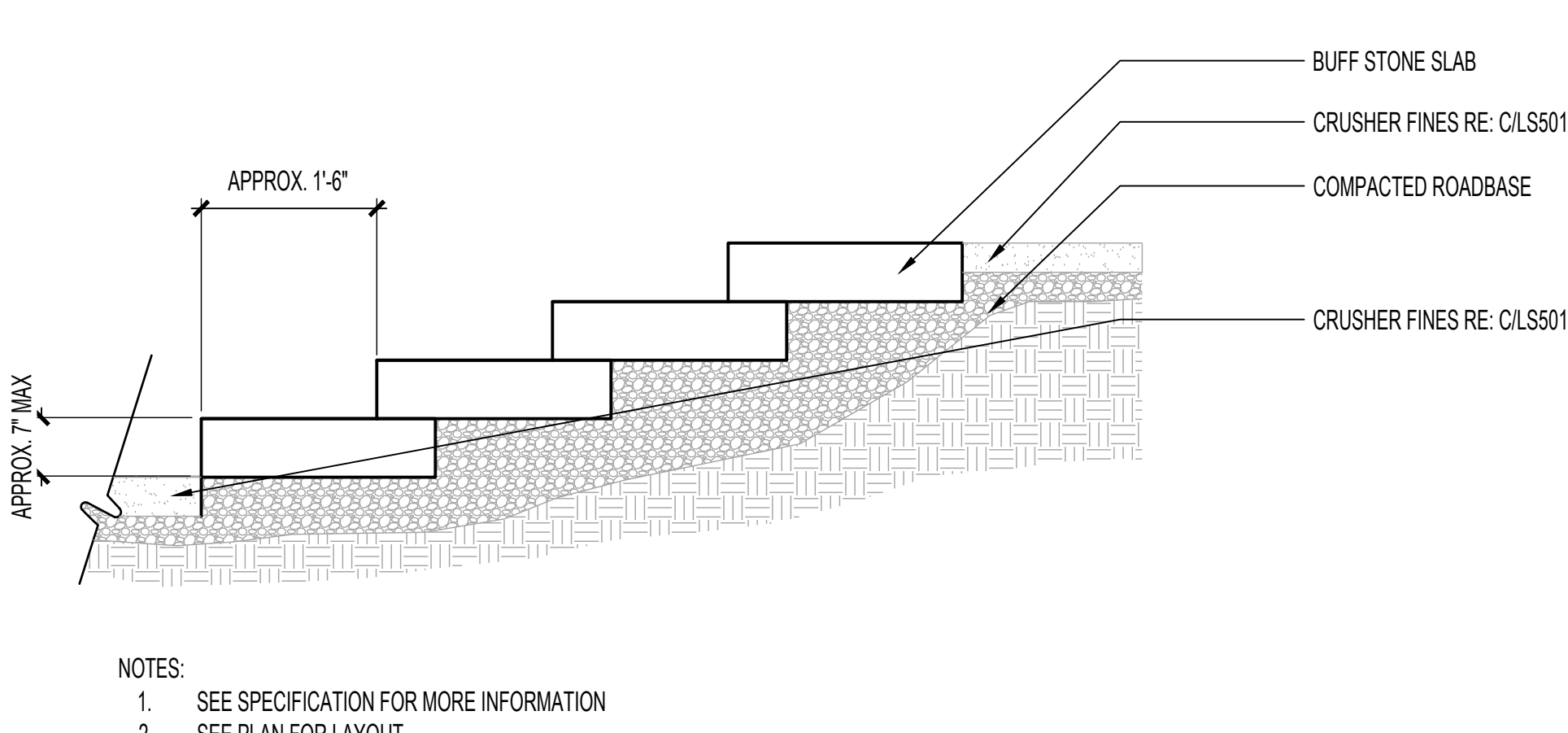
C SLAB STONE STEPS SCALE: 3/8" = 1'-0"
