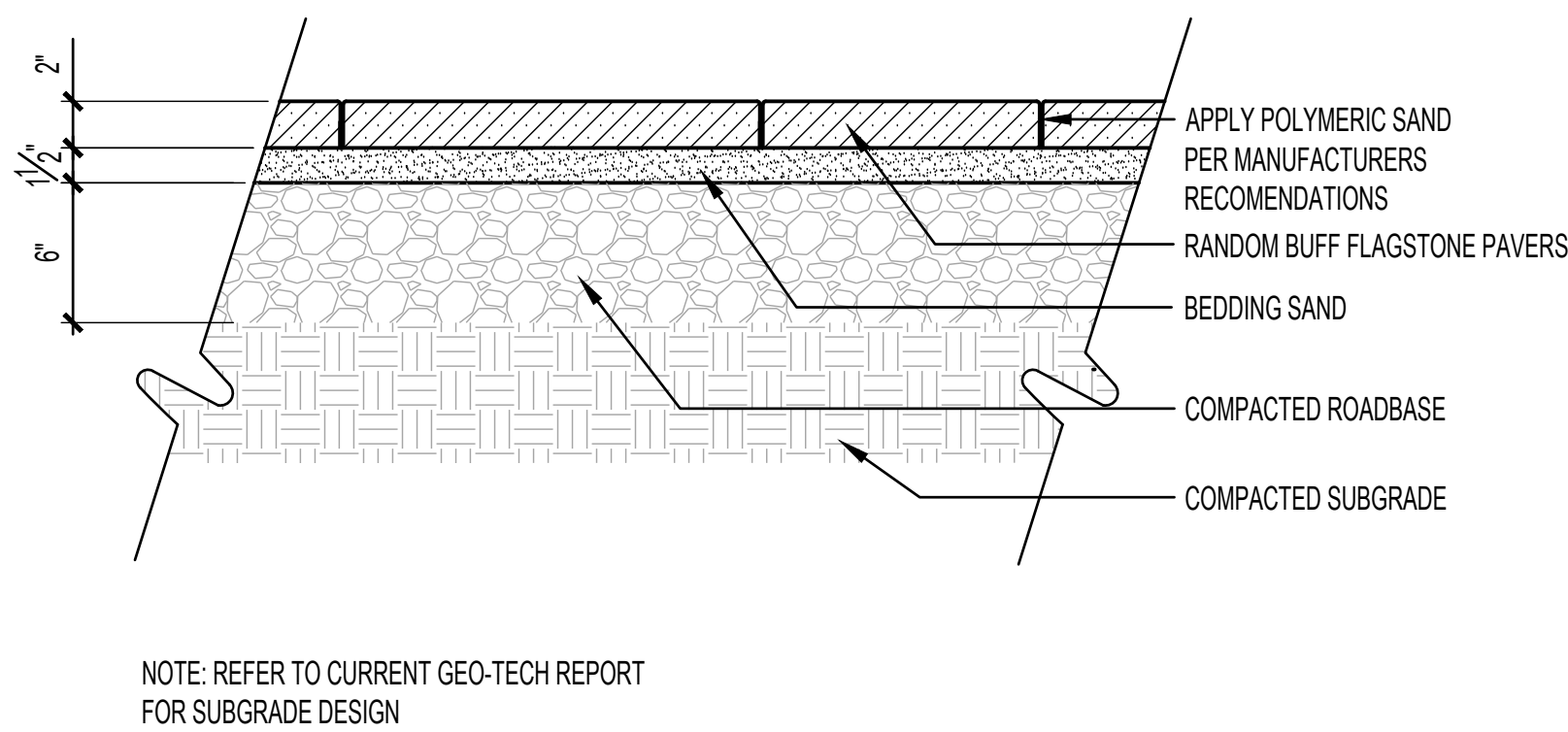
F FLAGSTONE PAVERS SCALE: 1/12" = 1'-0"
