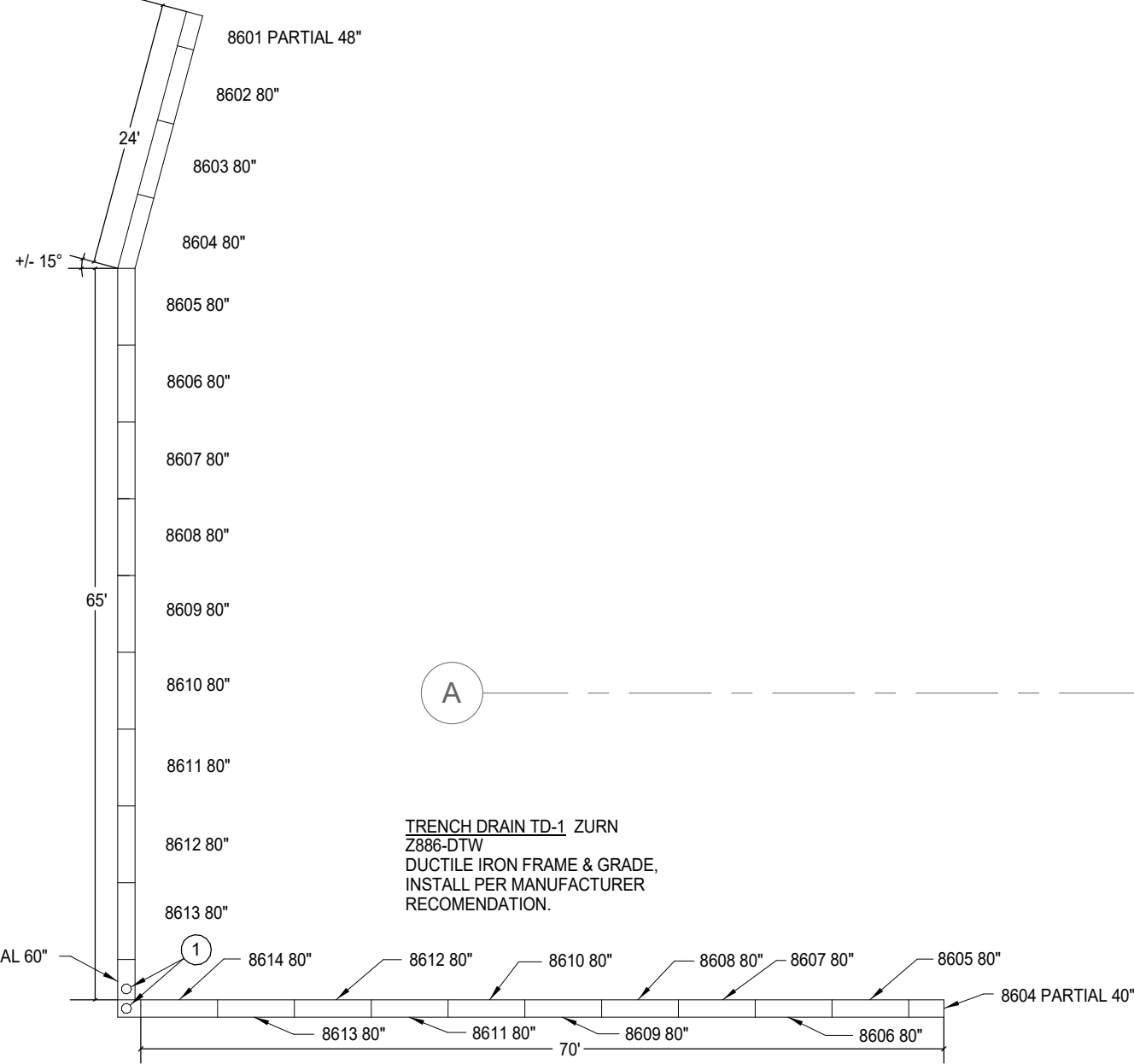
1 TRENCH DRAIN DETAIL SCALE: NONE
